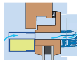
Figura 19d. EA ISOLA HY RA + viserilla acústica
