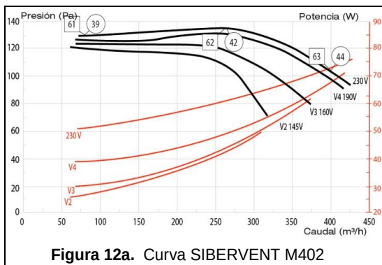
Figura 12. Curva característica Grupo Siber VMC SIBERVENT M
