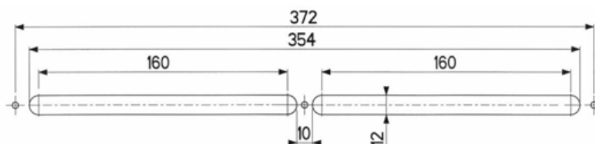
Figura 2. Dimensiones de las dobles ranuras para EA ISOLA HY (en mm)
