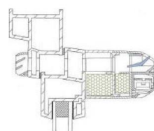
Figura 19c. EA ISOLA HY RA + viserilla estándar
