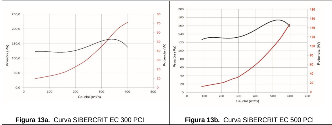
Figura 13. Curva característica Grupo SIBERCRIT EC
