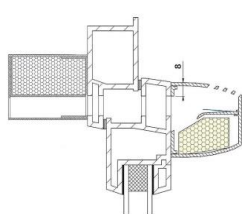
Figura 19a. EA ISOLA HY + viserilla estándar (mm)
