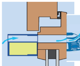
Figura 19b. EA ISOLA HY + viserilla acústica
