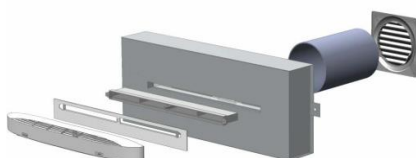
Figura 10. Vistas y despiece de las bocas de extracción
