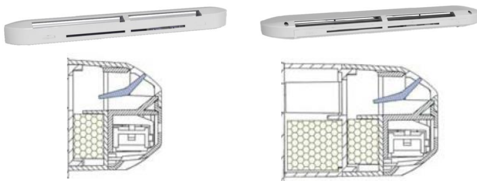
Figura 1a. EA ISOLA HY
