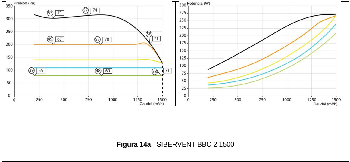
Figura 14. Curva característica Grupo Siber VMC SIBERVENT BBC 2
