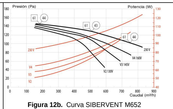
Figura 12. Curva característica Grupo Siber VMC SIBERVENT M
