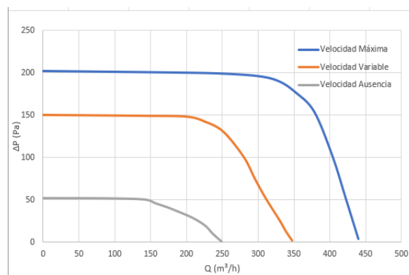
Figura 17. Curva característica Grupo ECO HIGRO+
