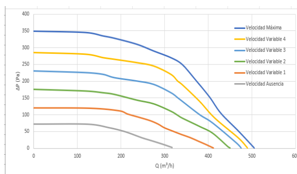
Figura 17. Curva característica Grupo ECO HIGRO+
