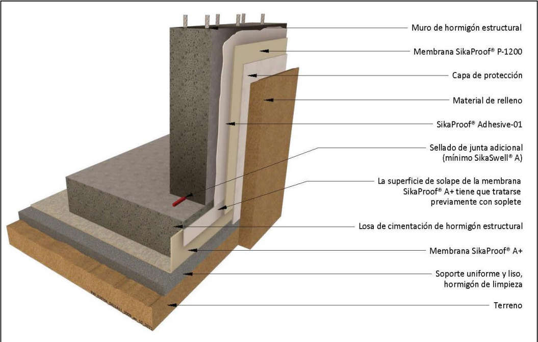
Fig. 11. SikaProof® A+ Conexión losa de cimentación. Con sistema pre aplicado en losa SikaProof® A+ y post aplicado en muro SikaProof® P-1201
