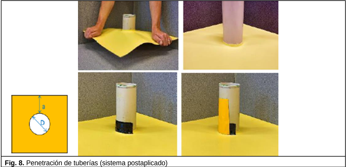
Fig. 8. Penetración de tuberías (sistema postaplicado)
