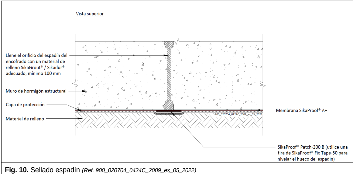
Fig. 10. Sellado espadín (Ref. 900_020704_0424C_2009_es_05_2022)
